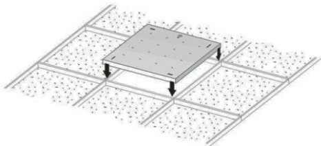
Рисунок 7 — Установка светильника Geniled серии Офис на подвесную конструкцию.
